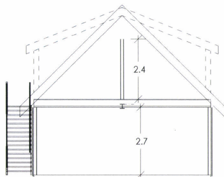
SNITT A-A
