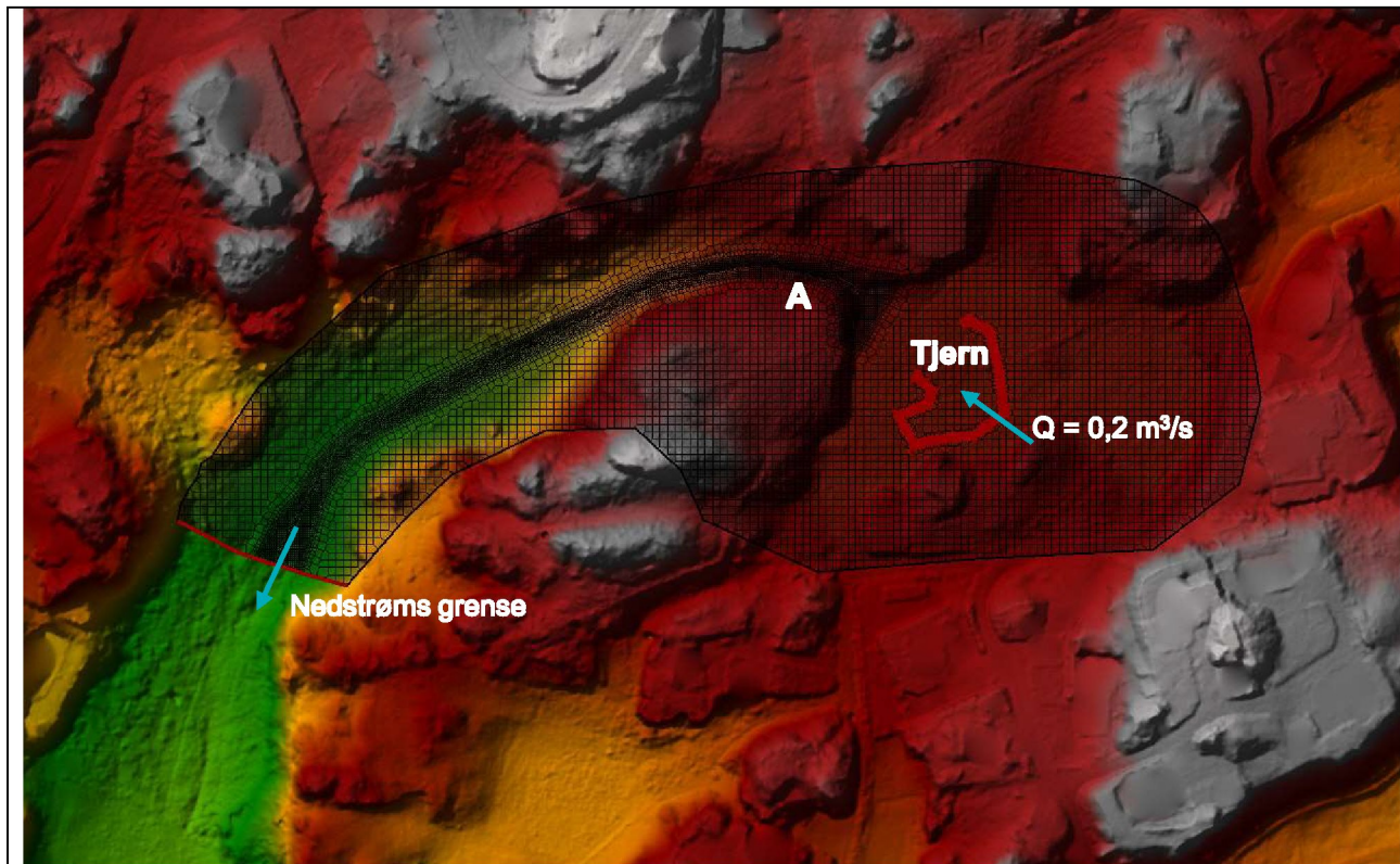
Figur 8: Høydemodell over modellert område.
