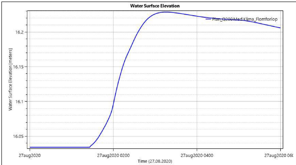
Figur 10: Simulerte vannstander i tjernet.
