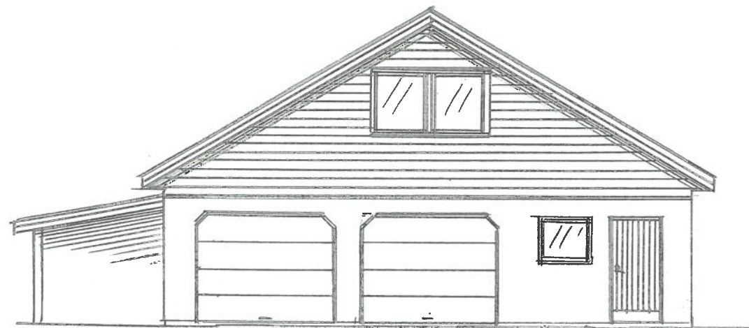
FASADE SØR
