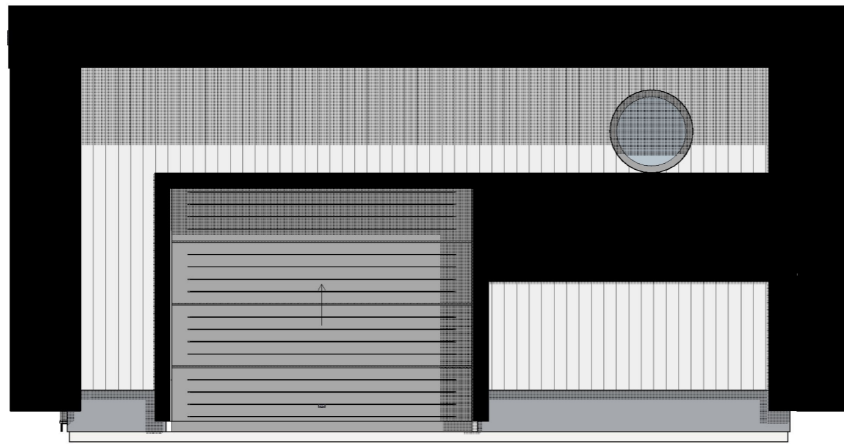
1:50 Fasade-Nord
