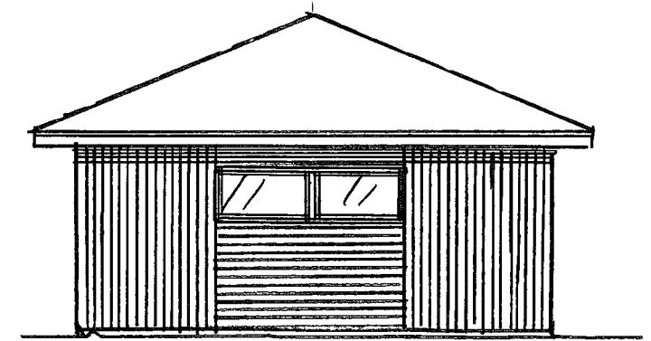
FASADE VEST
