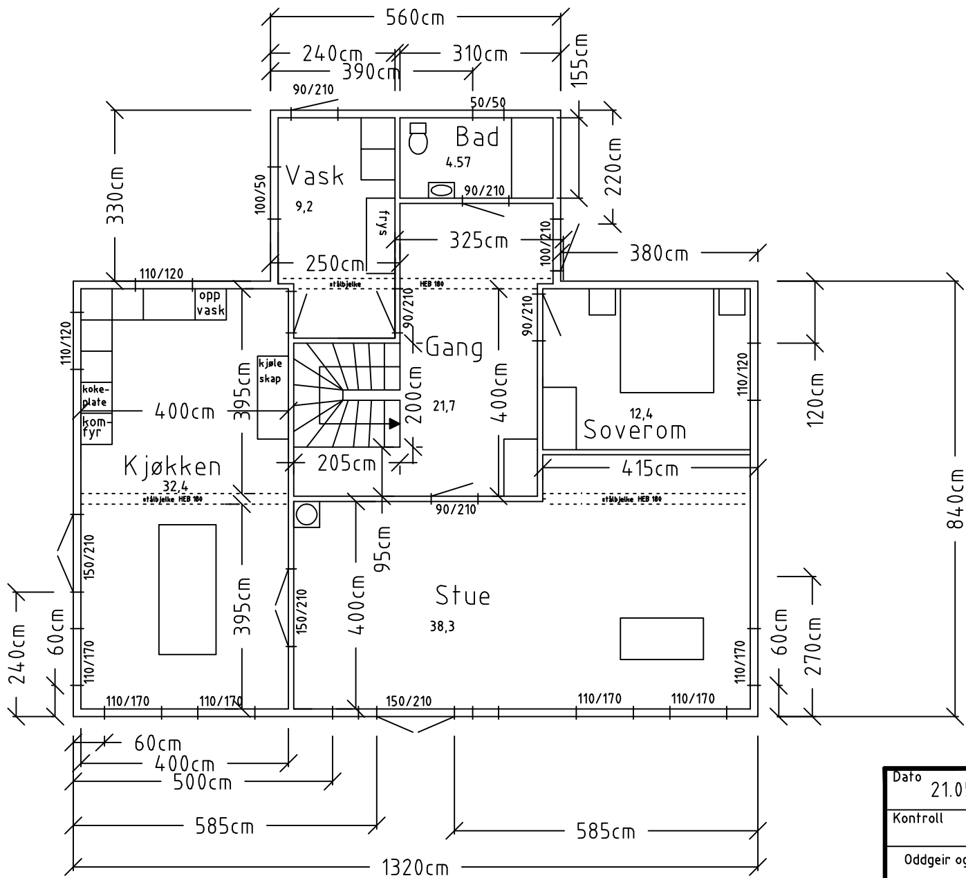
Plan hovedplan
