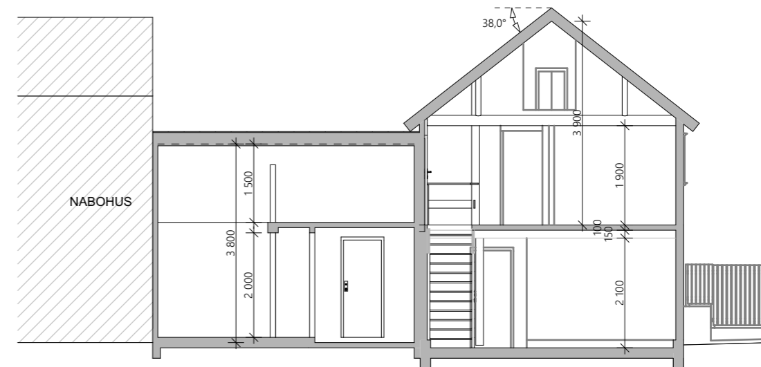
SNITT B
