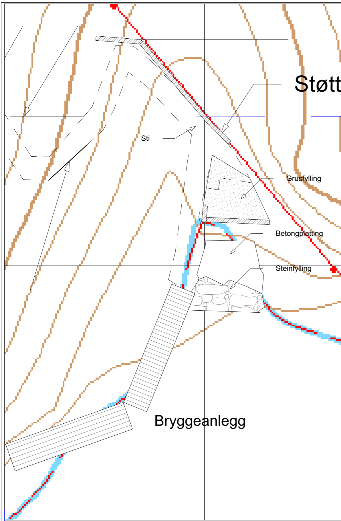
Utsnitt-situasjonskart-bryggeanlegg 1:100
