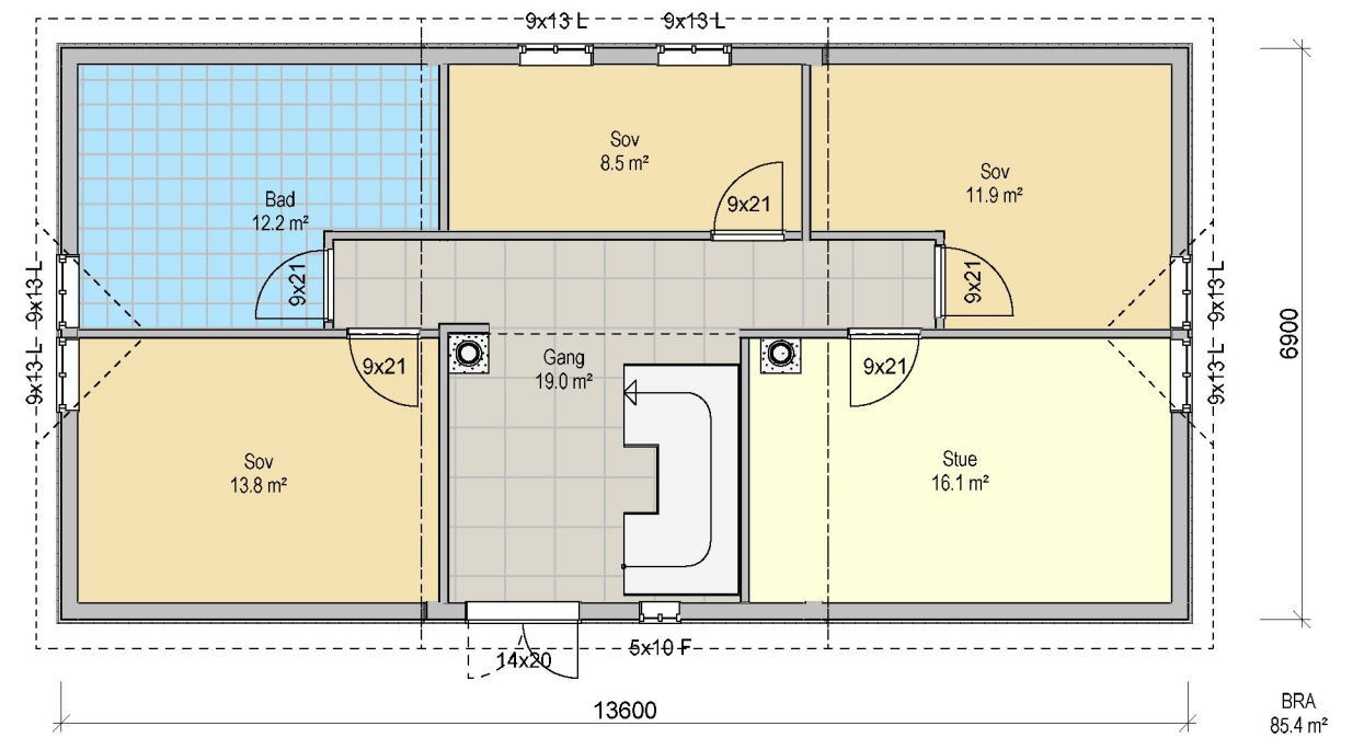
Plan 2 etg
