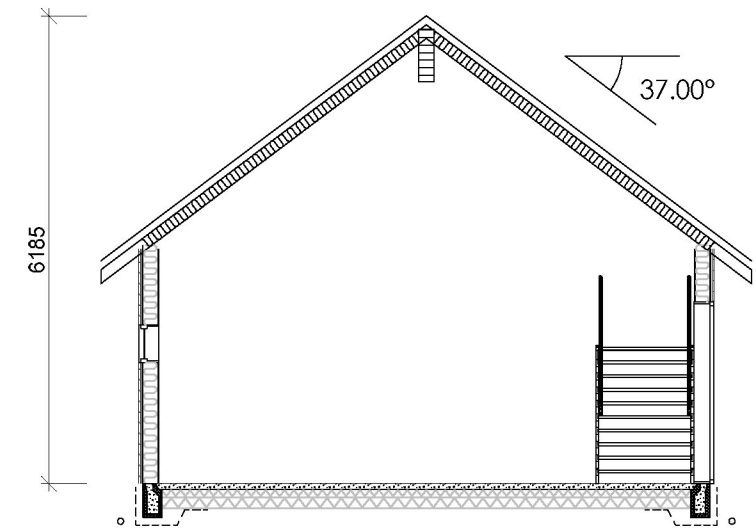
Snitt B:B
