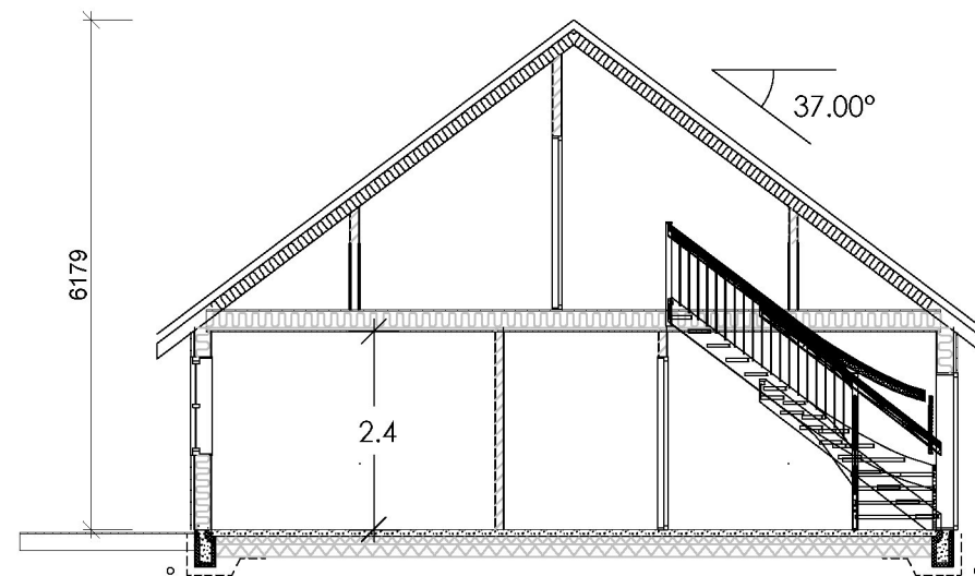
Snitt A:A
