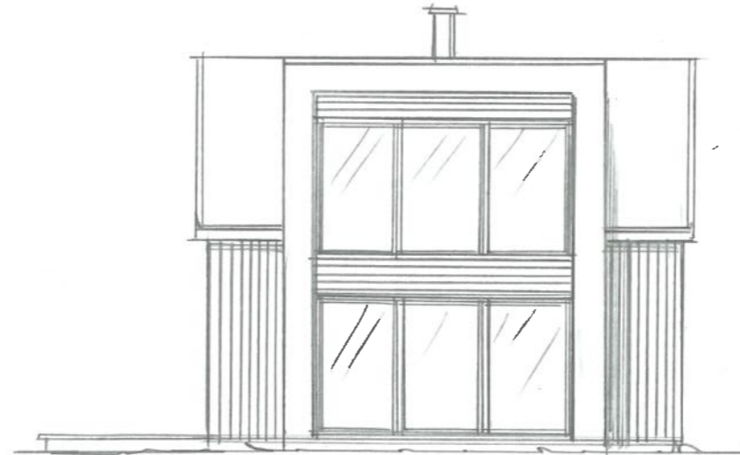
FASADE ØST
