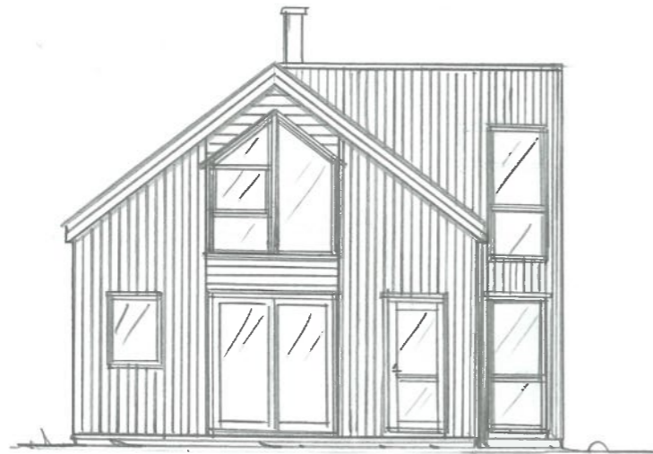
FASADE SØR
