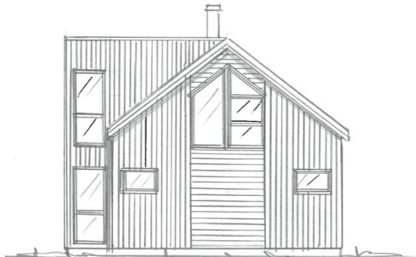
FASADE NORD
