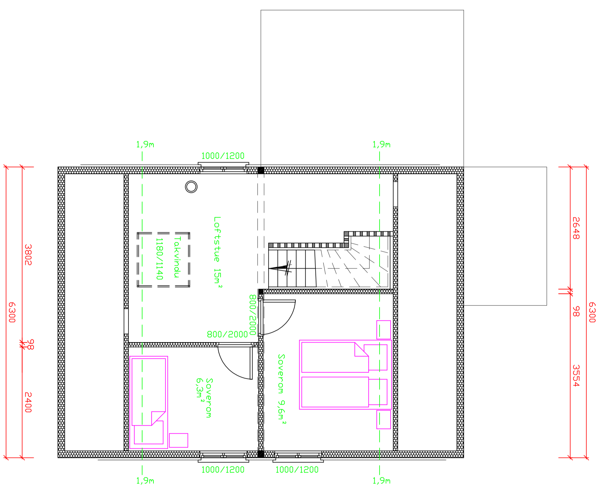
Plantegning lofetasje
