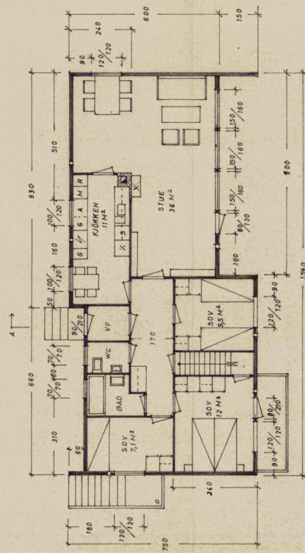
1. ETASJE
