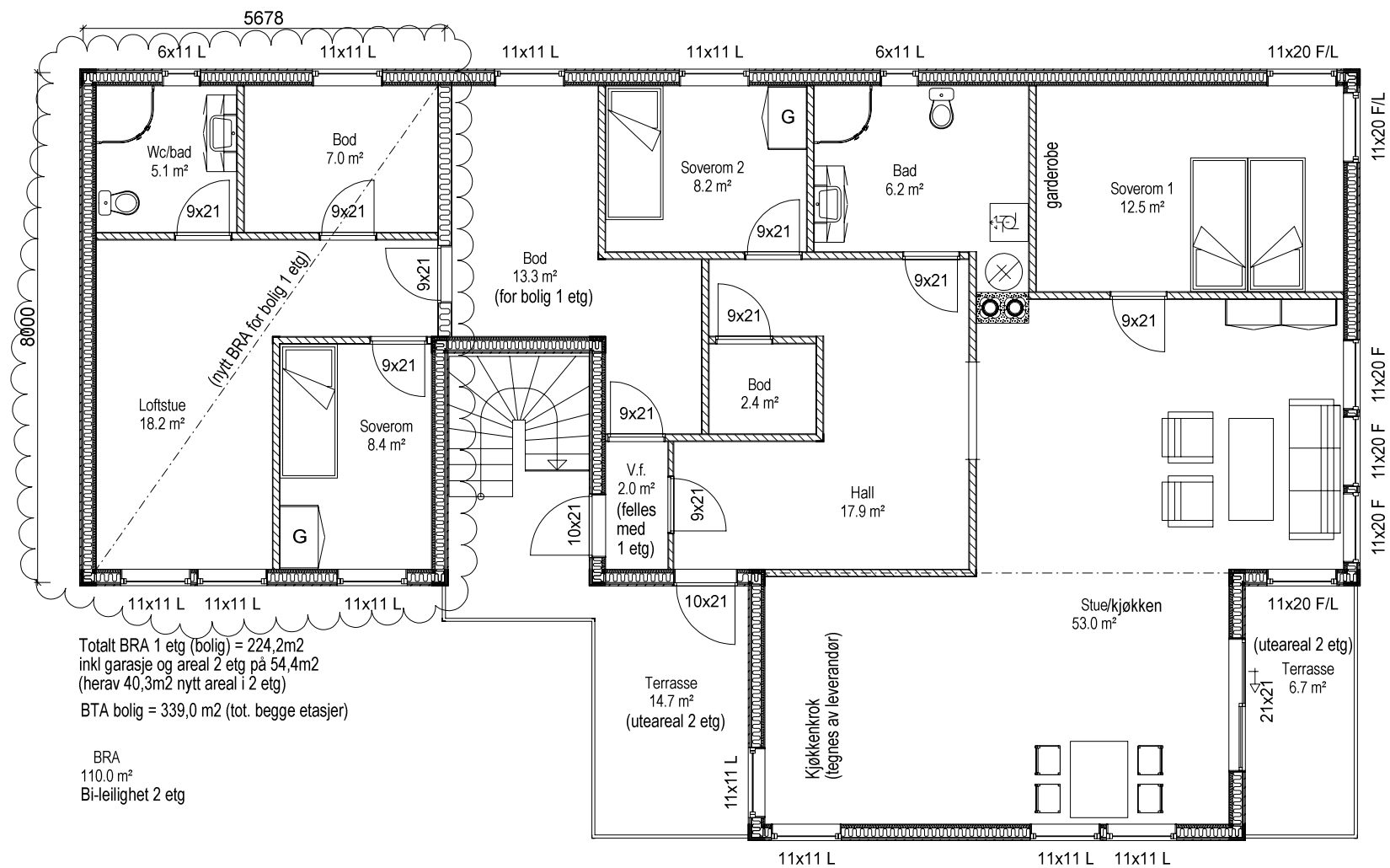
Plan 2 etg
