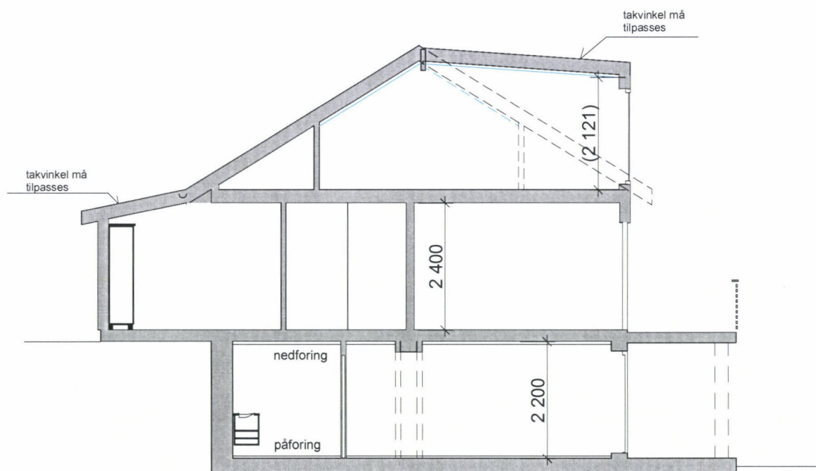
1:100 Snitt B
