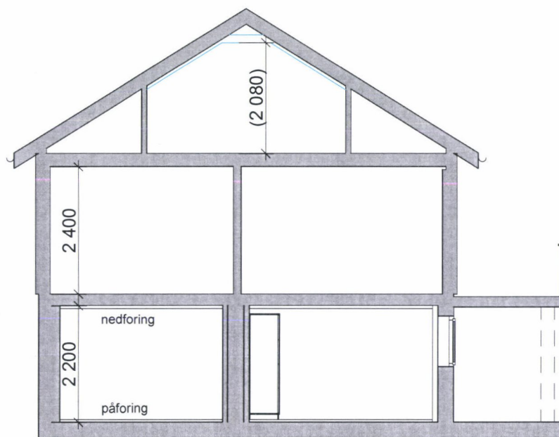
1:100 Snitt A
