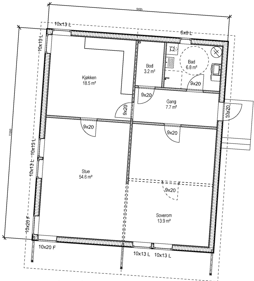
Hovedplan (boligdel)
