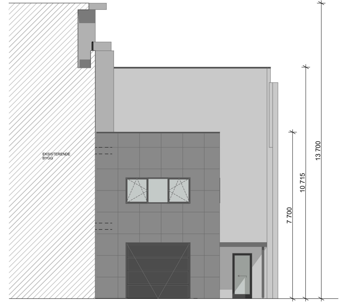
FASADE SØR
