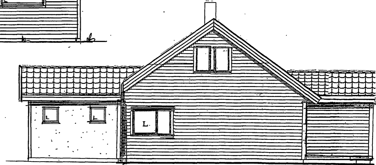
Tilbygg FASADE MOT NORD
