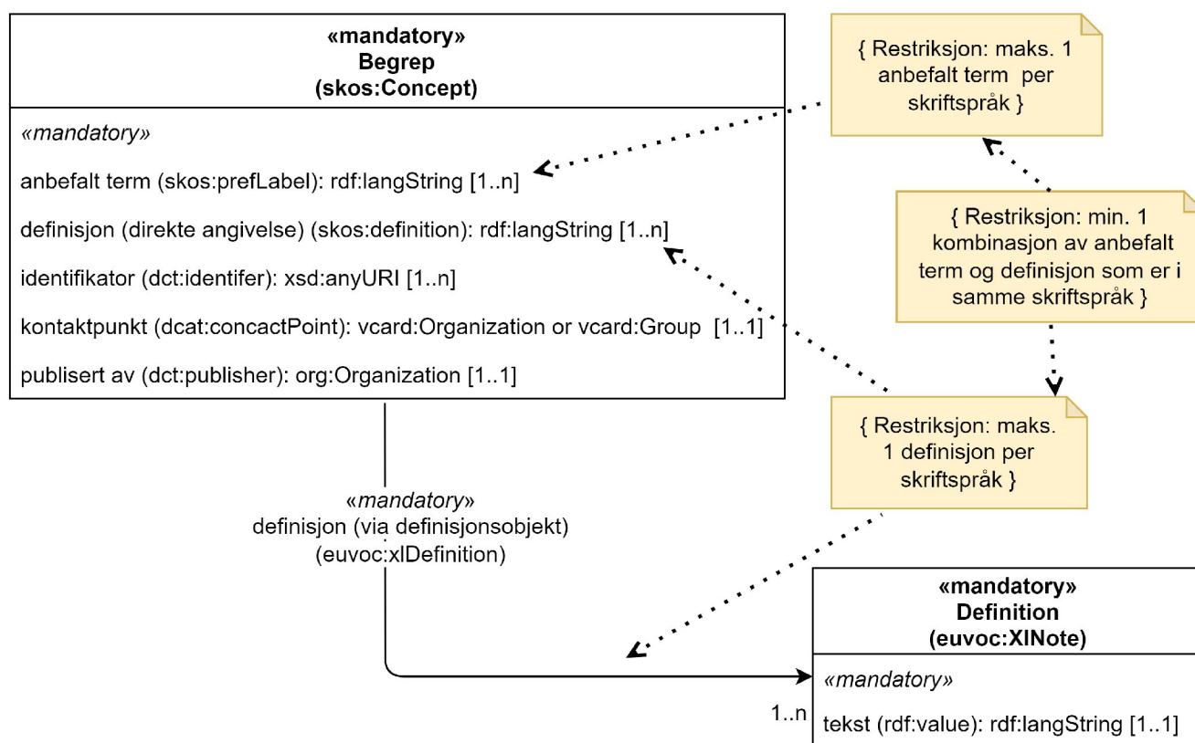
Figur 5. Forenklet modell for SKOS-AP-NO-Begrep, med kun obligatoriske klasser og deres obligatoriske egenskaper. Se beskrivelse av den enkelte egenskapen for mer detaljert beskrivelse av restriksjonene.
