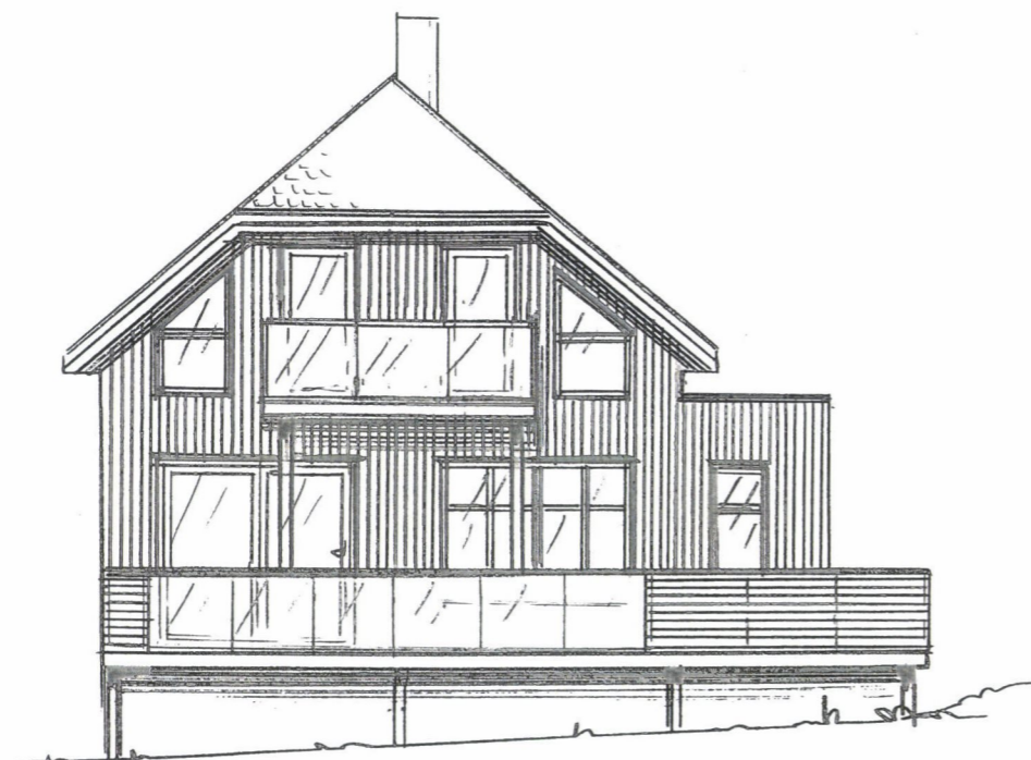
FASADE SØR-ØST
