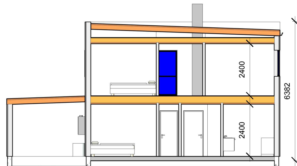
Section 2 1 : 100
