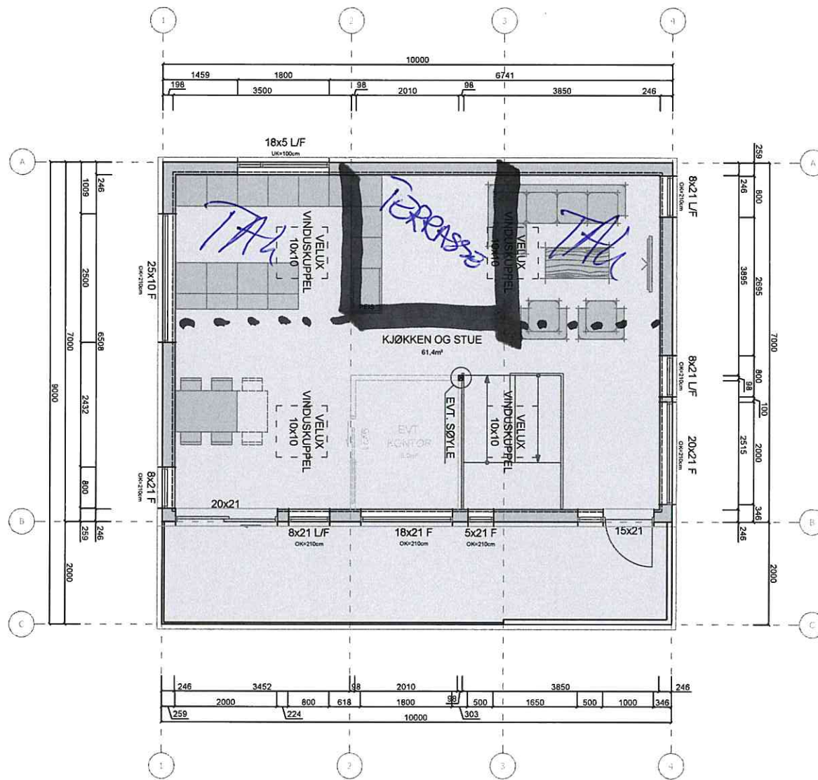
PLAN 3. ETASJE
