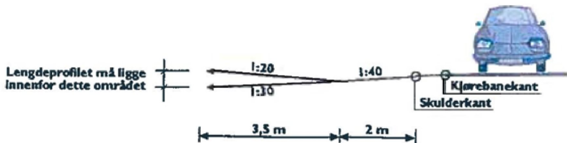
Figur 2: Lengdeprofil
