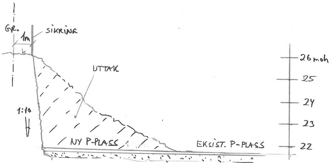
SNITT 1:100
