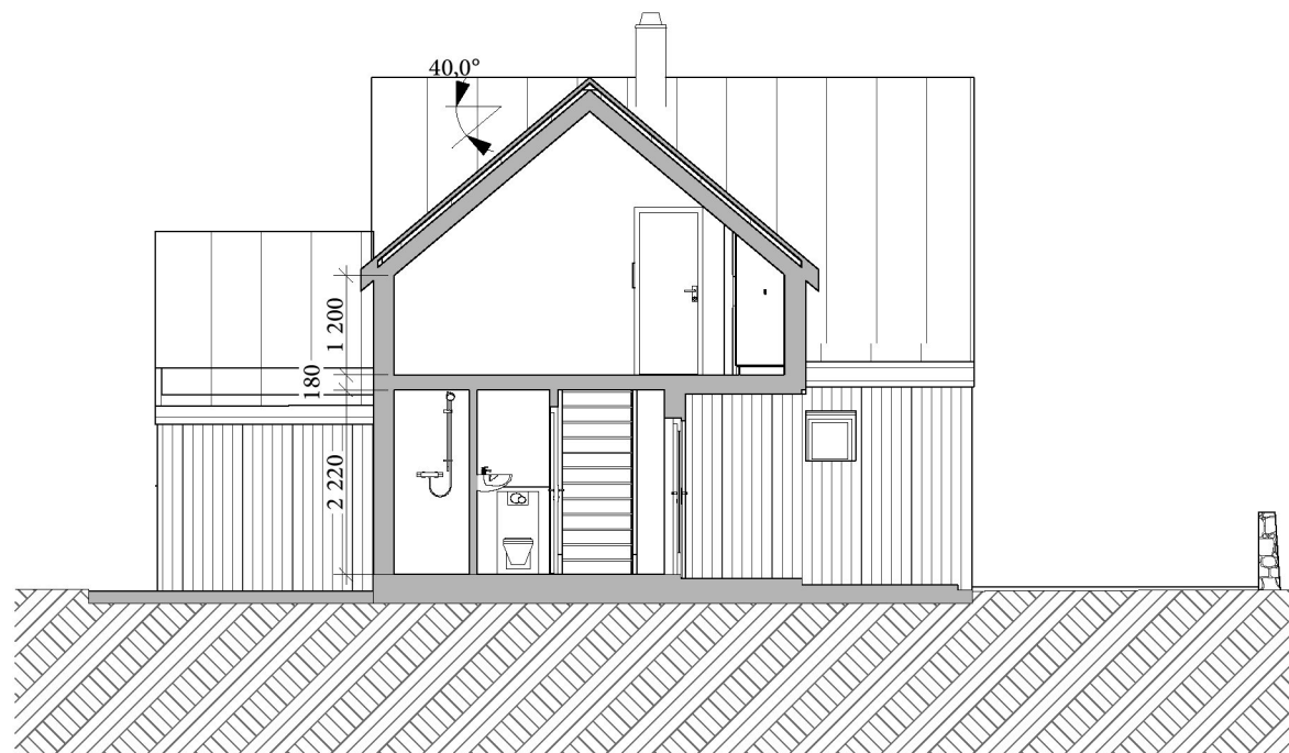
SNITT A-A
