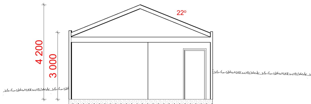
snitt garasje
