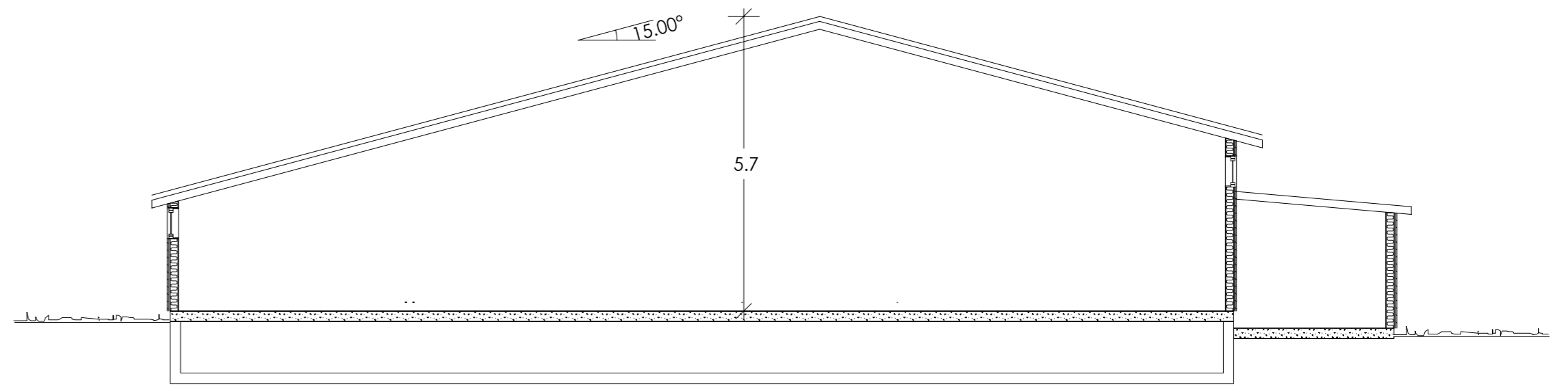
Snitt A-A
