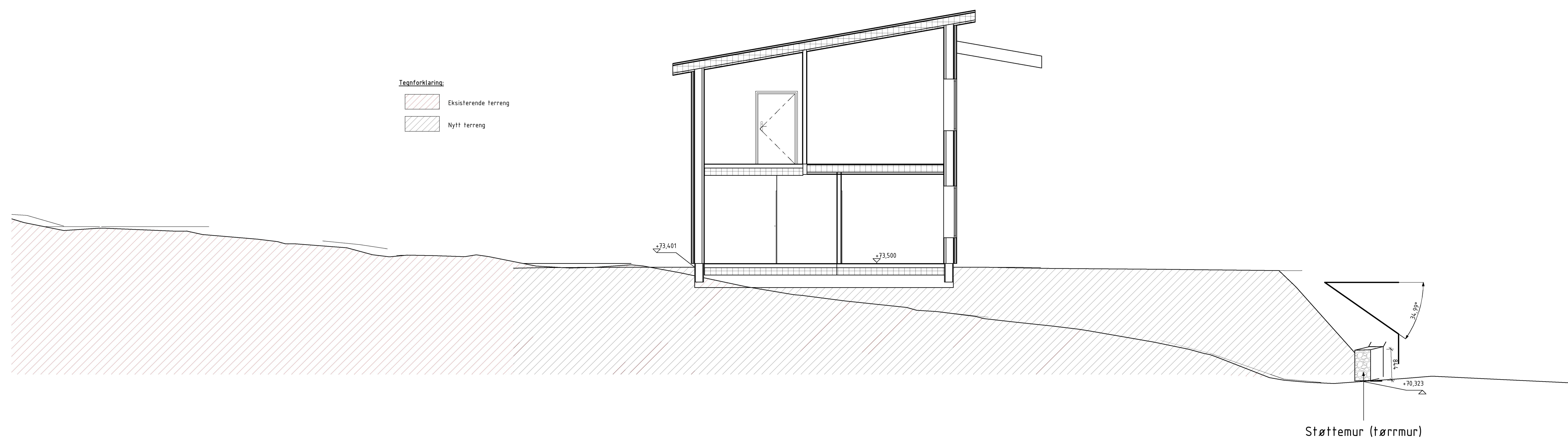
Terrengsnitt 1 1 : 50
