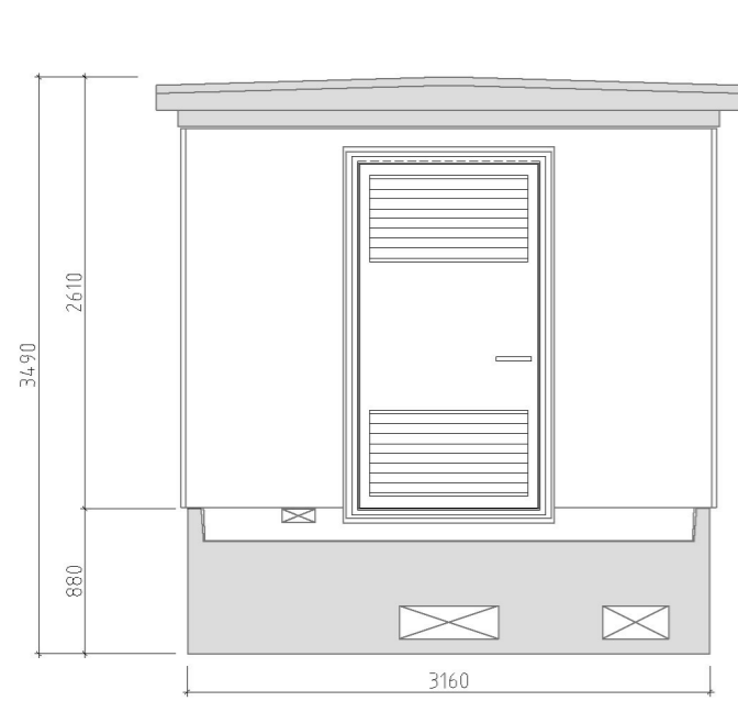
FASADE VEST
