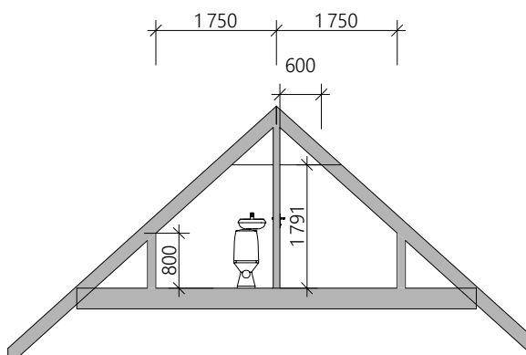
Snitt A
