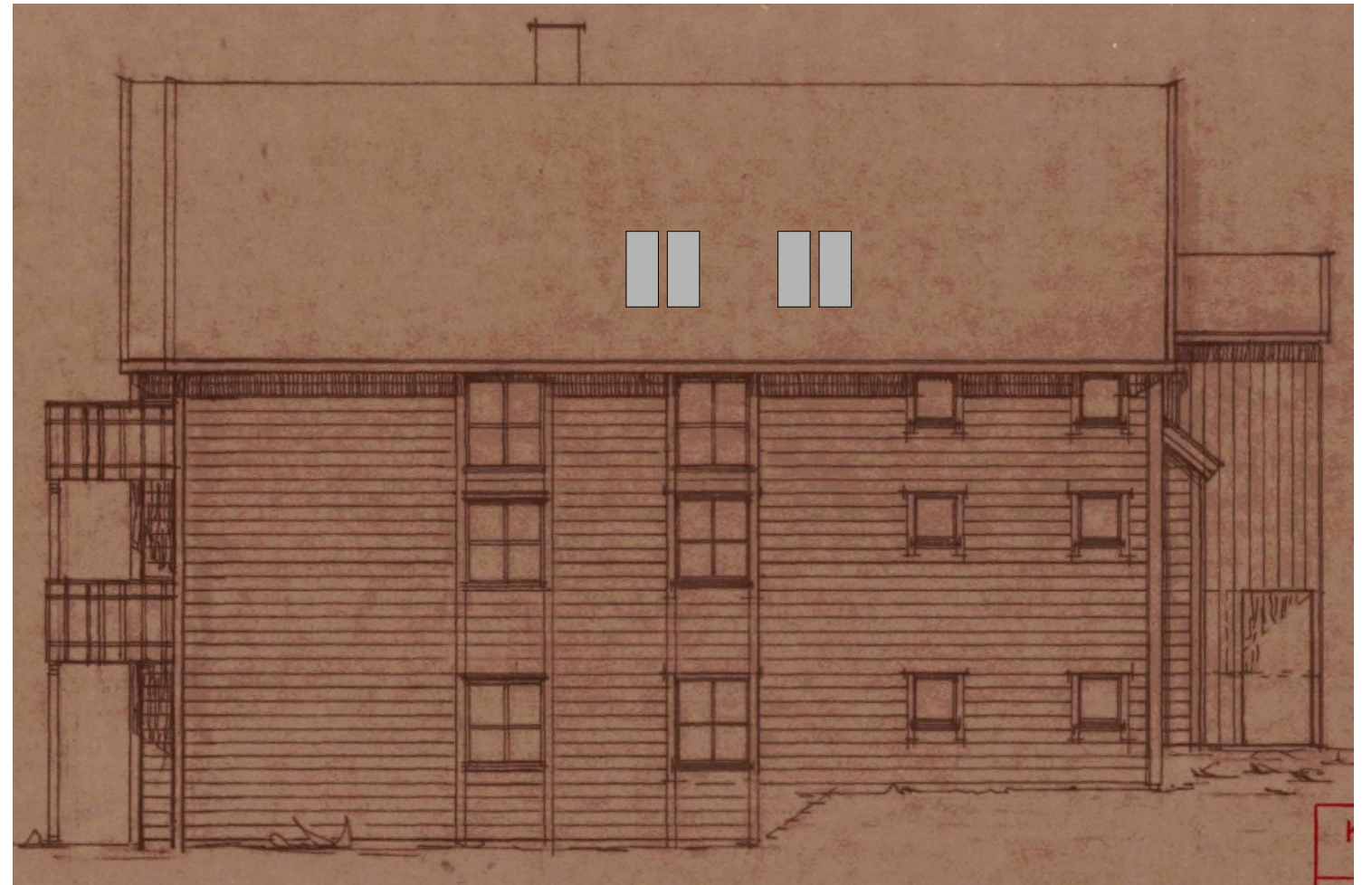
1:100 Fasade Sør
