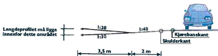
Figur 2: Lengdeprofil
