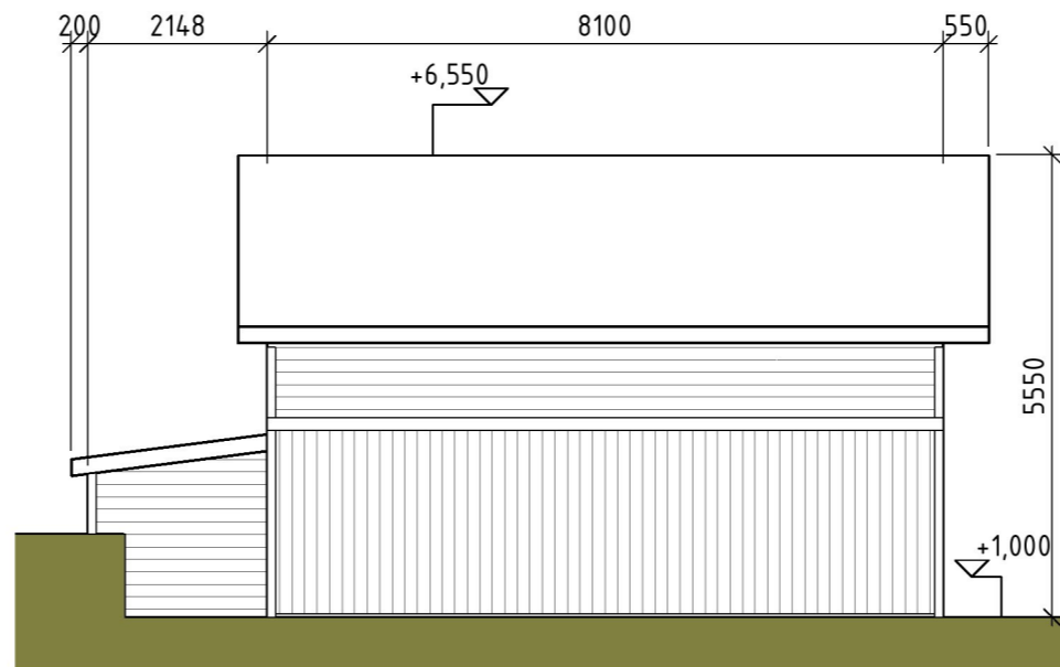
Fasade nordvest 1 : 100
