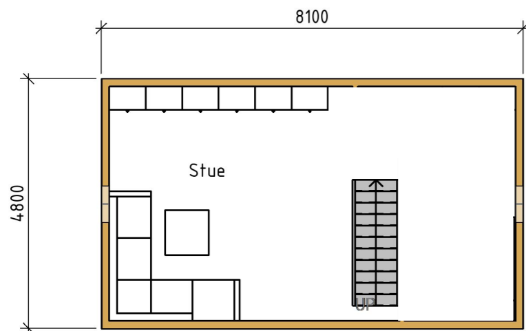
Plan loft 1 : 100
