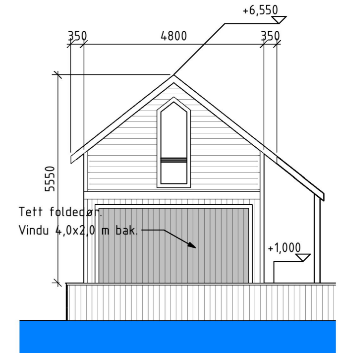
Fasade sørvest 1 : 100
