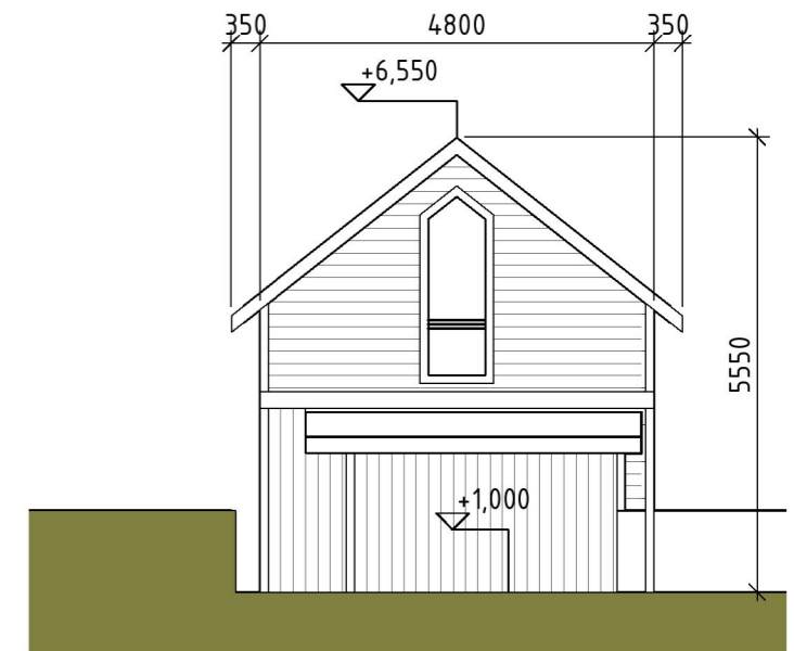
Fasade nordøst 1 : 100
