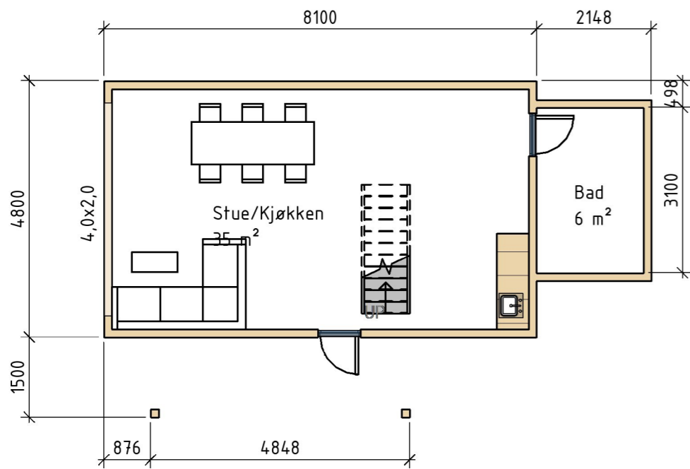
Plan 1.etg 1 : 100
