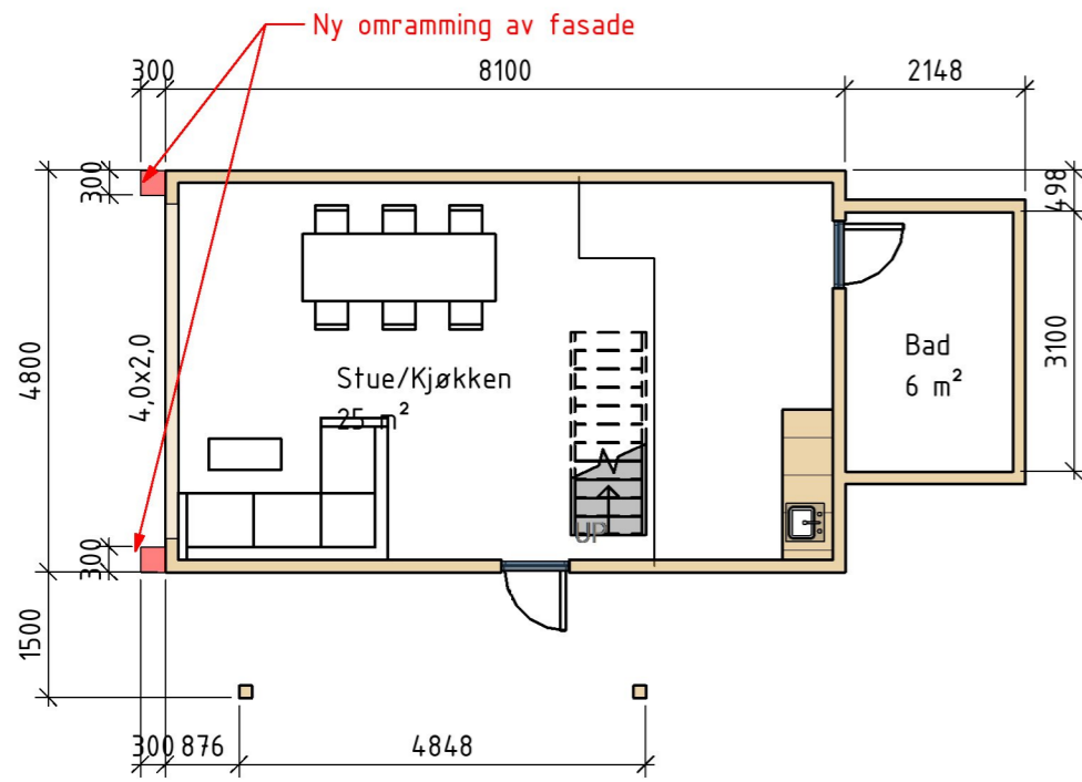
Plan 1.etg 1 : 100
