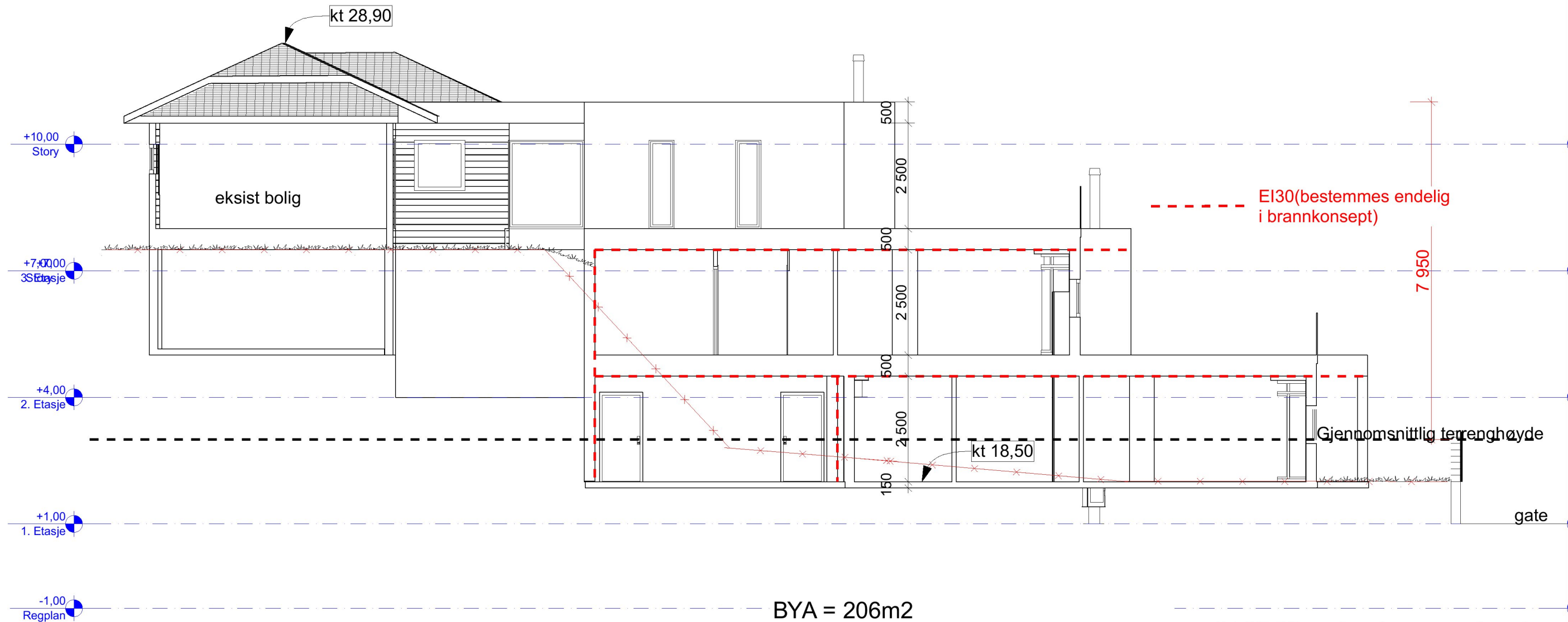
1:100 Snitt B
