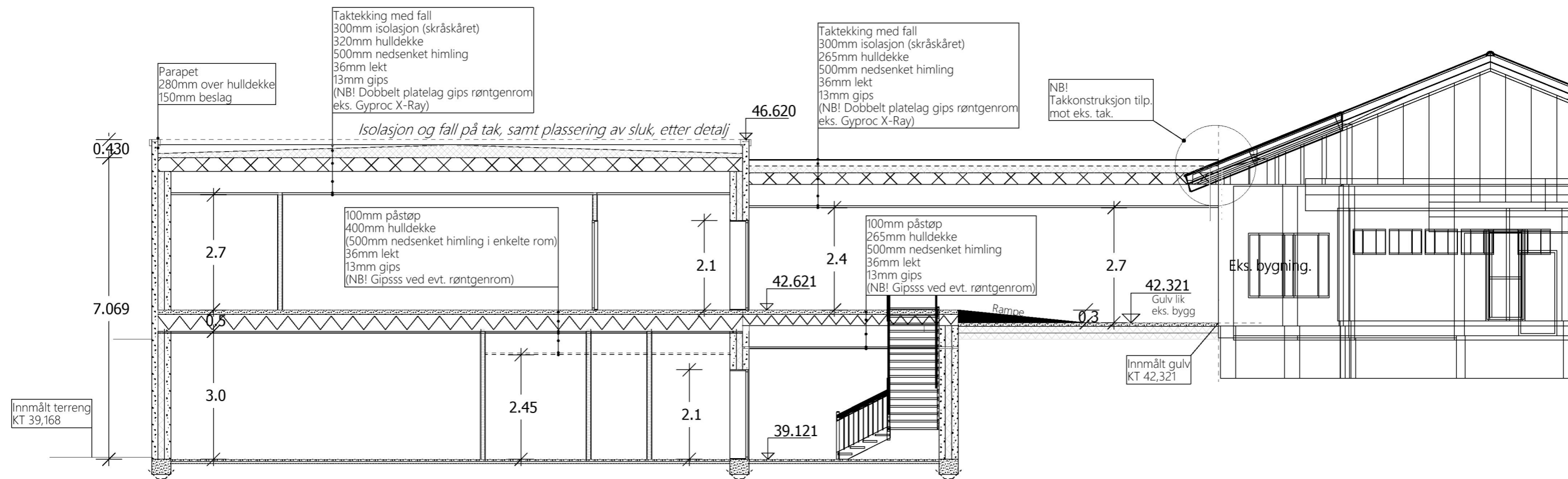
Snitt A-A
