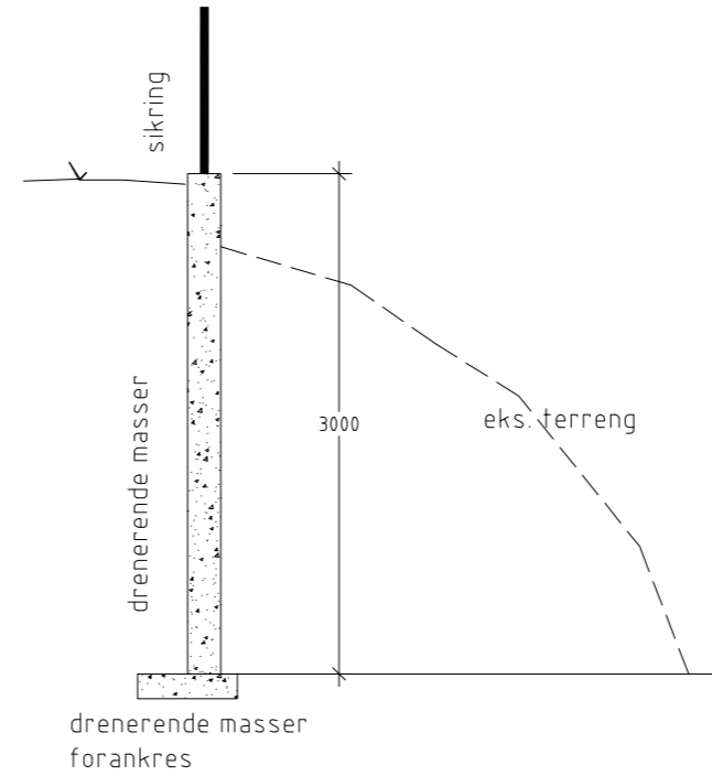
SNITT PROFIL 1 1:50
