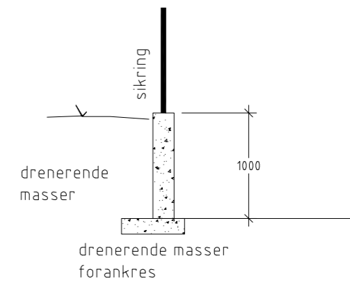
SNITT PROFIL 2 1:50
