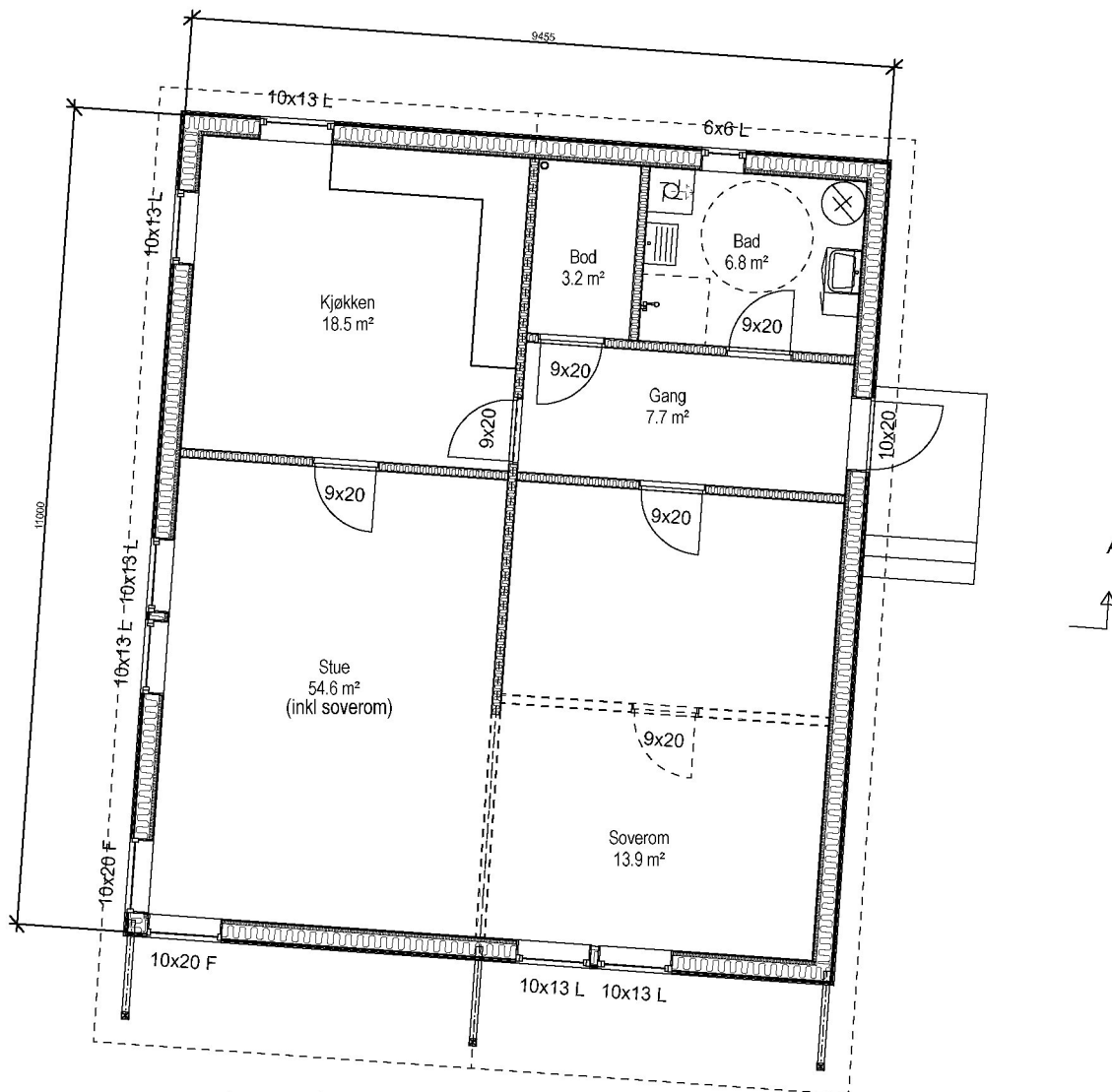
Hovedplan (boligdel)
