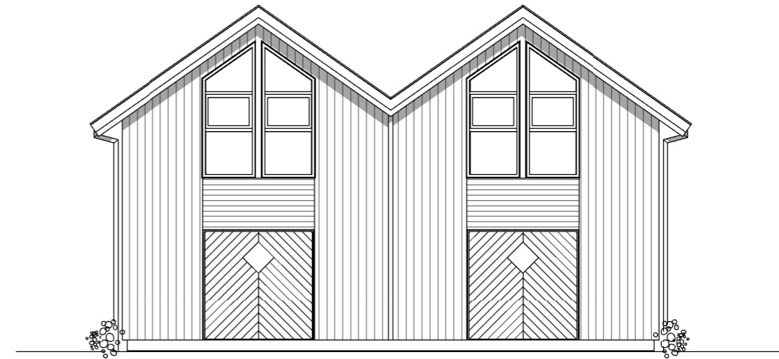
Fasade mot nord 1 : 100
