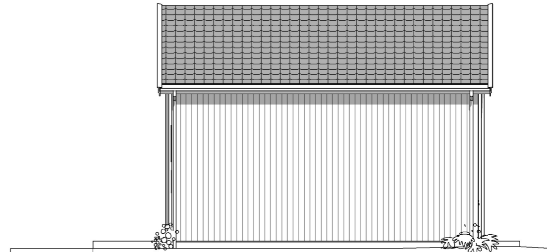
Fasade mot vest 1 : 100
