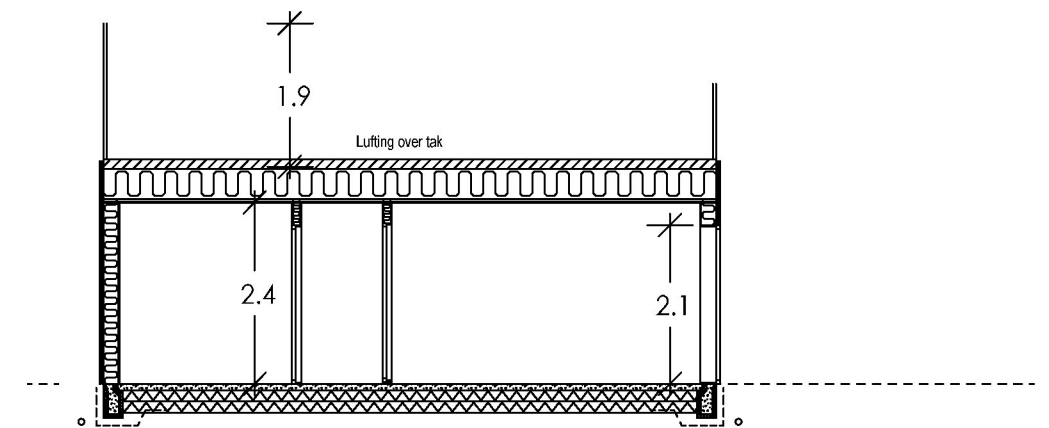
Snitt B:B
