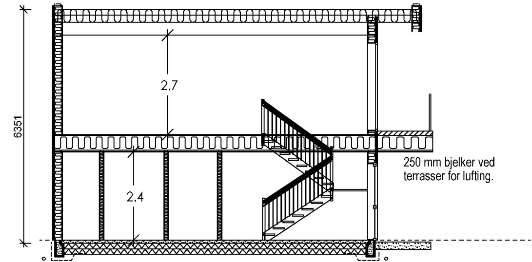
Snitt A:A
