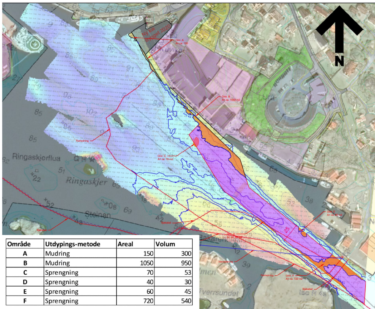
Figur 1 Planlagt utdyping av eksisterende innseiling. Mudring er markert med lilla. Sprengning er markert med oransje. Kilde: Petter J. Rasmussen AS
