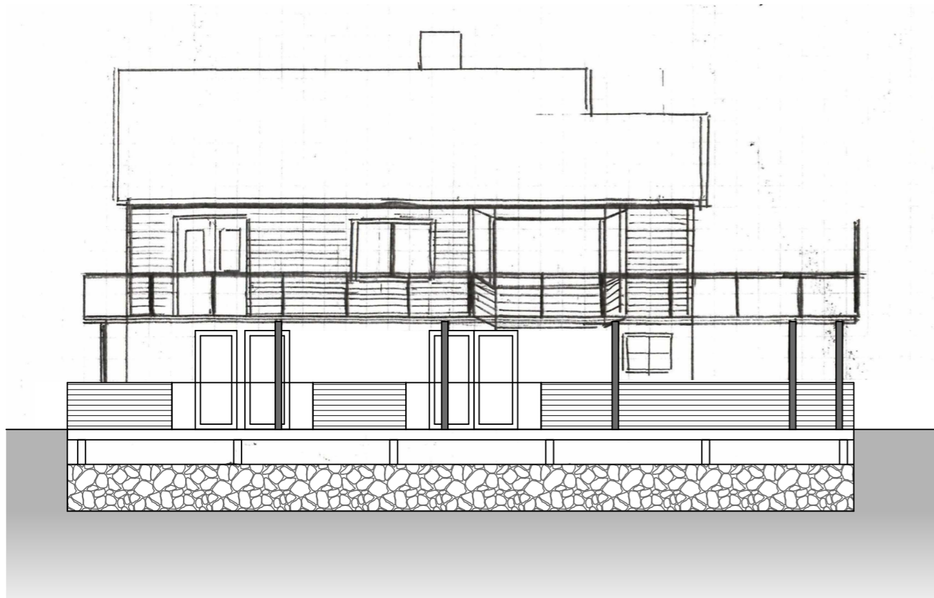
FASADE VEST
