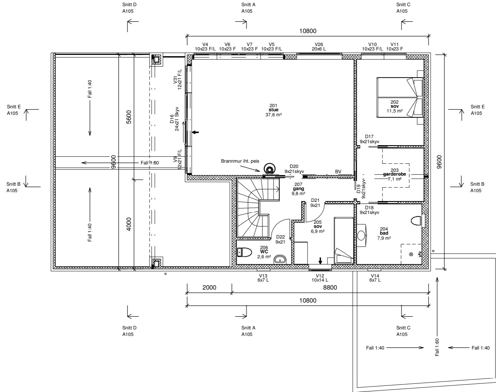
2.0 - 2.etasje 1 : 100
