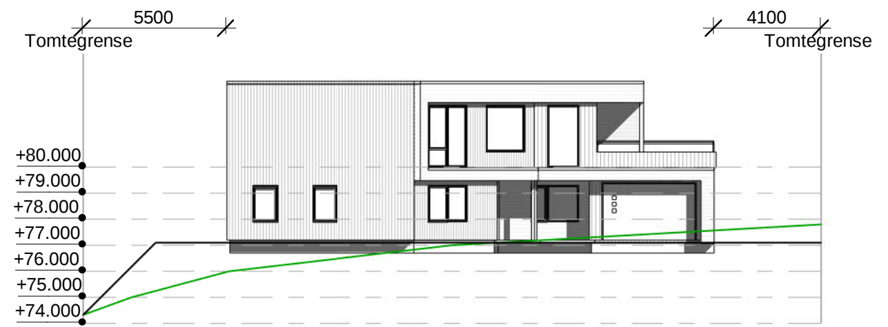
Terrengsnitt Nord 1 : 200
