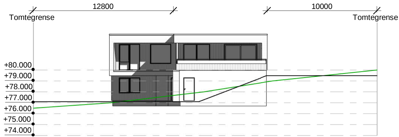
Terrengsnitt Vest 1 : 200
