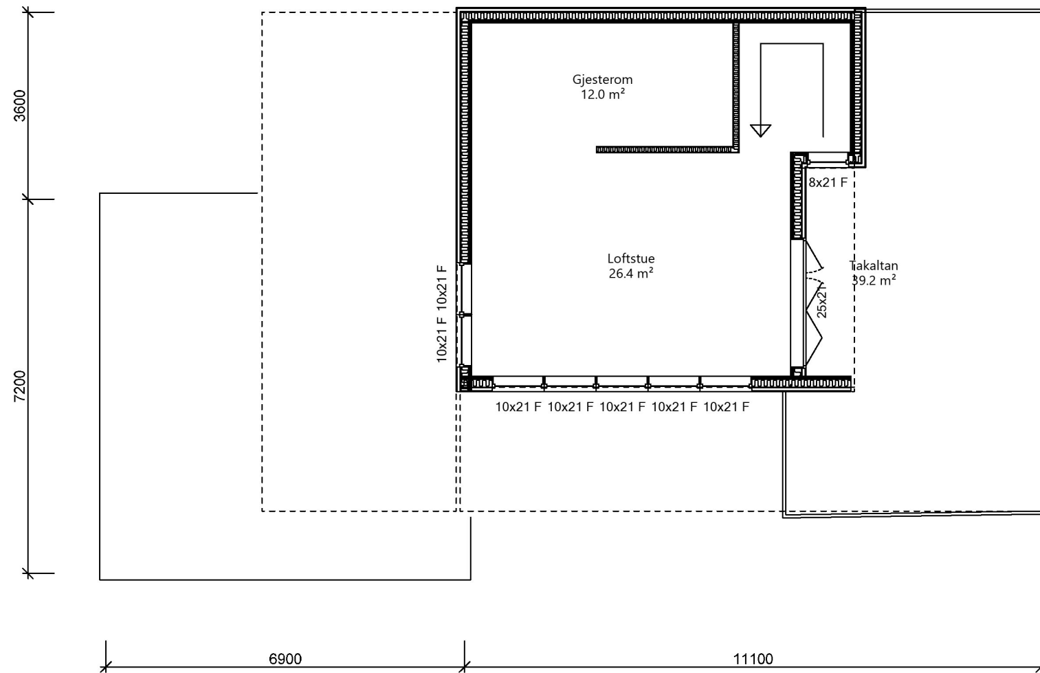
Plan 3.etg
