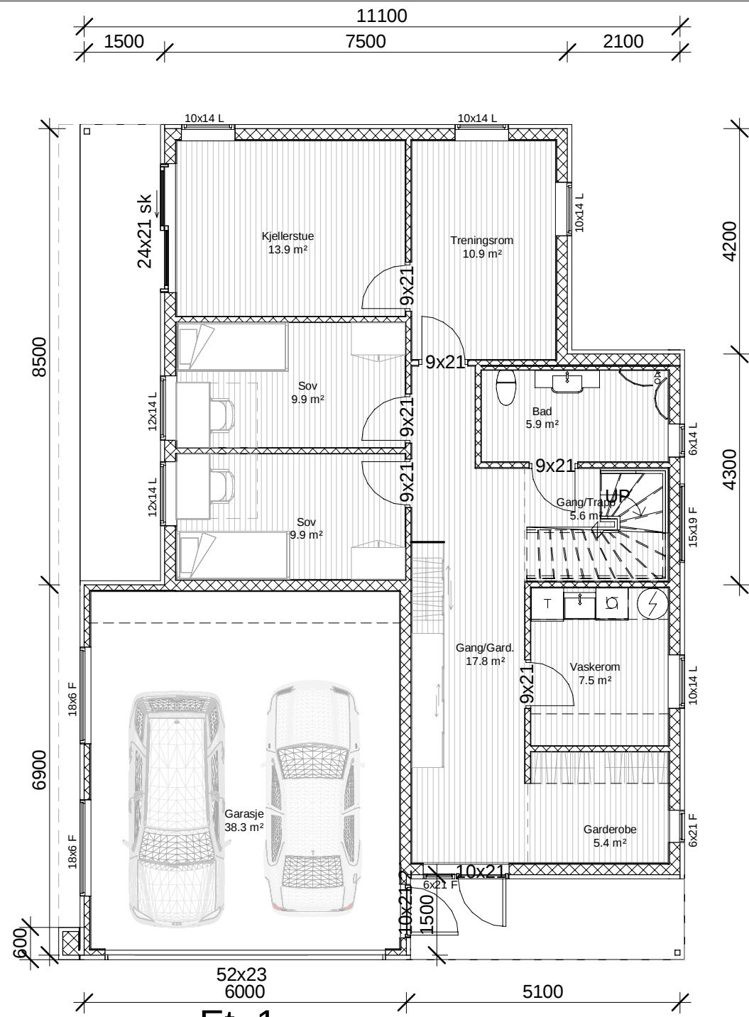
Et. 1 1 : 100
