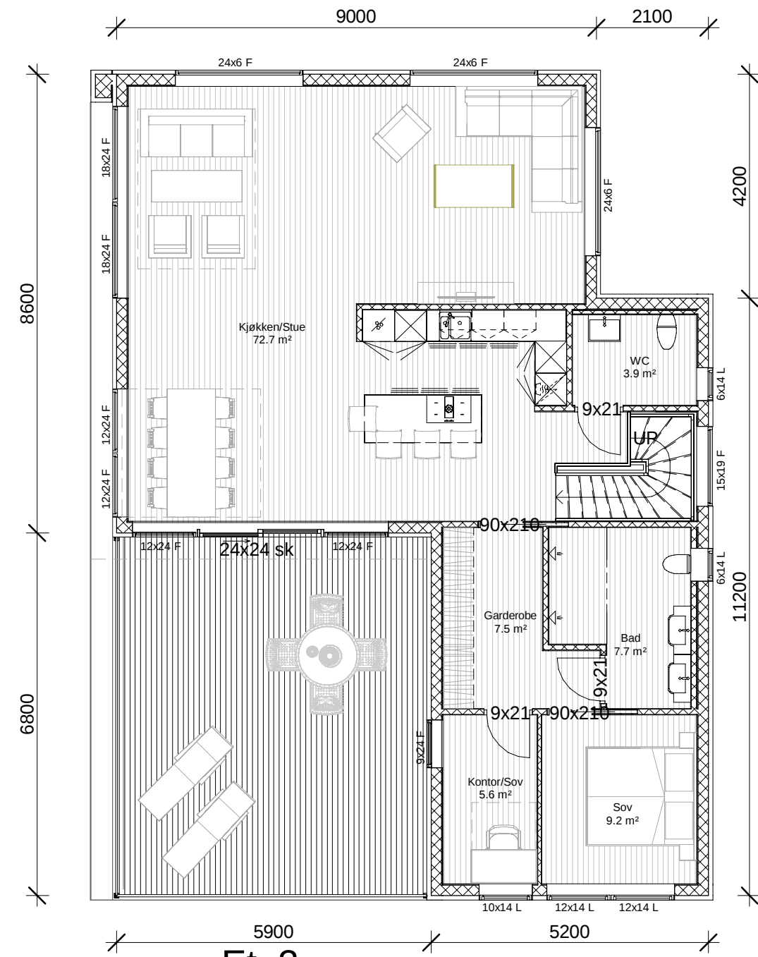
Et. 2 1 : 100
