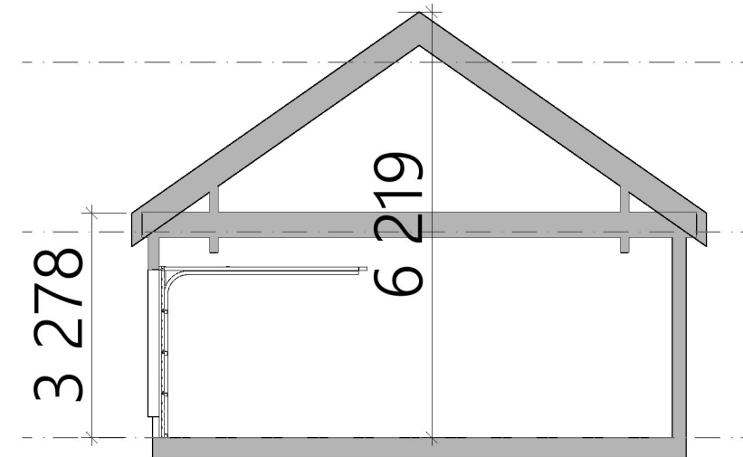
1:100 Snitt B
