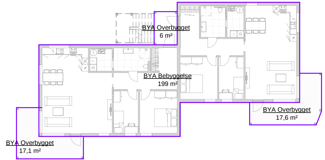
Et. 1 1 : 200
