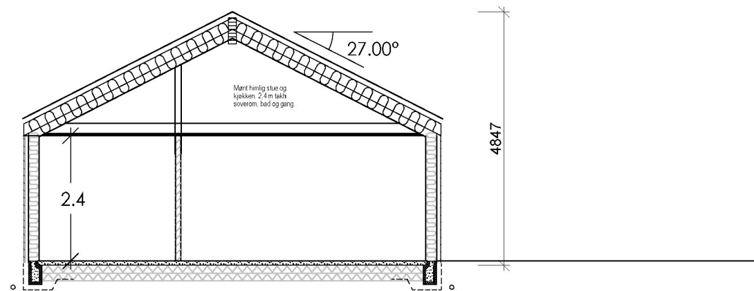
Snitt A:A
