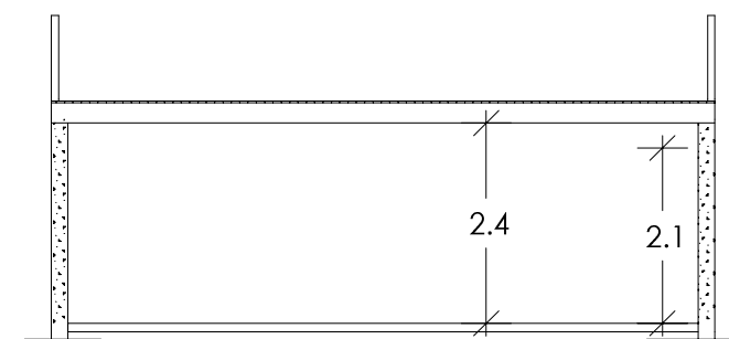
Snitt garasje
